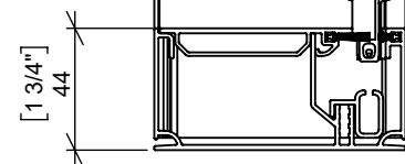
SECTION A-A SCALE 1 : 3
