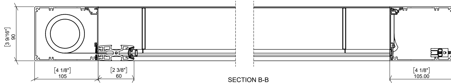
SECTION B-B SCALE 1 : 3
