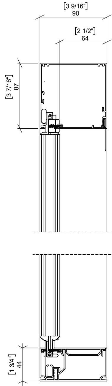
SECTION A-A SCALE 1 : 3
