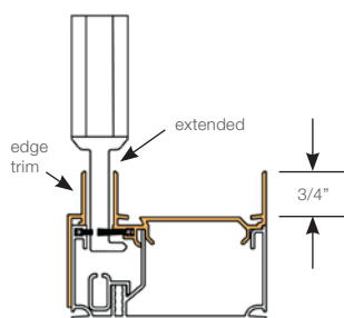
S4 Invisible sill
